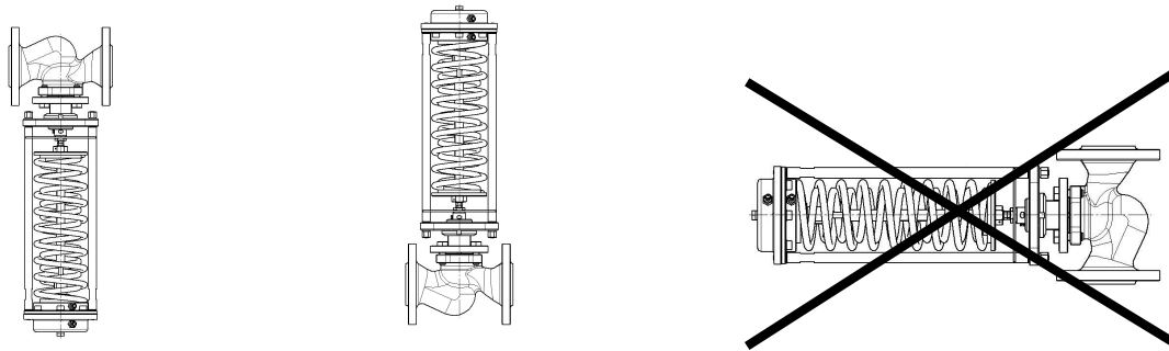
Рисунок А.3-Монтажные положения регулятора на трубопроводе при температуре среды до 100 °С
