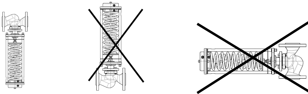
Рисунок А.4-Монтажные положения регулятора на трубопроводе при температуре среды выше 100 °С
