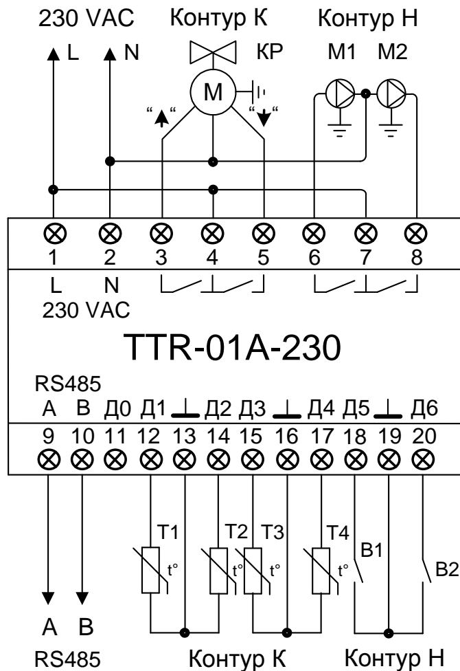
Рисунок В.1 - Схема электрическая подключений TTR-01A-230
